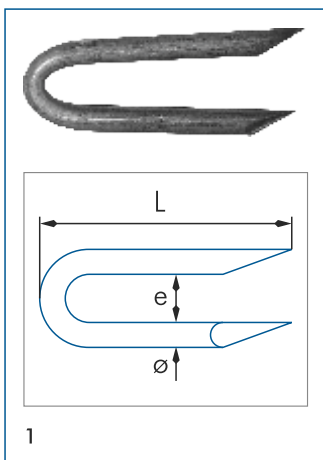
Schlaufen nach DIN 1159, Abb. 1
