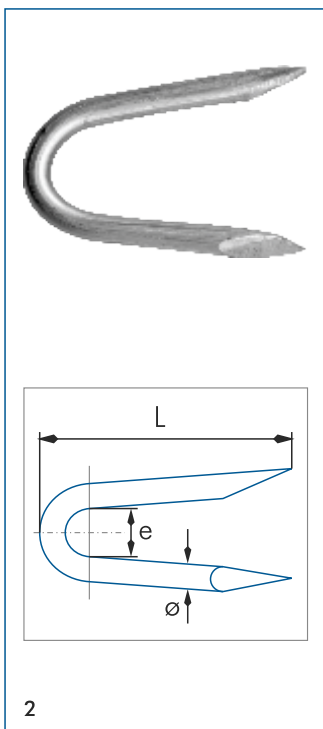
Krampen, Abb. 2
